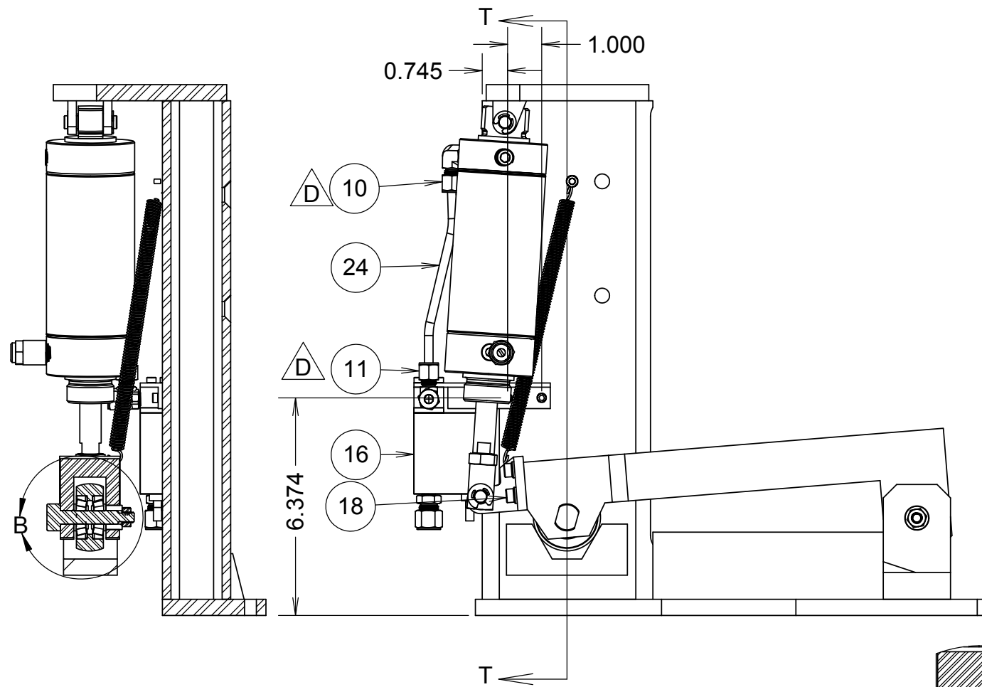
SECTION T-T SCALE 1 : 4
