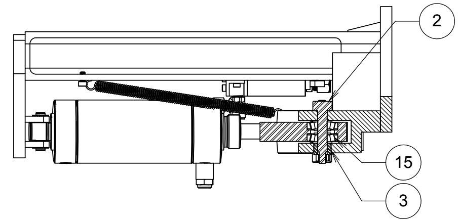
SECTION A-A SCALE 1 : 4
